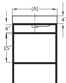
Round basin with apron and free standing frame codes Codes de cadre sur pied et bassin rond avec tablier
