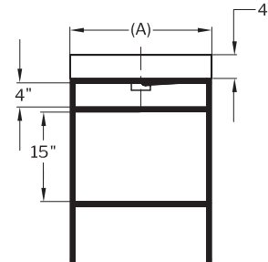
Square basin with apron and free standing frame codes Codes de cadre sur pied et bassin carré avec tablier
