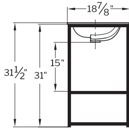
Round basin without apron and free standing frame codes Codes du bassin rond sans tablier et cadre sur pied
