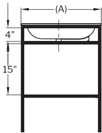
Round basin without apron and free standing frame codes Codes du bassin rond sans tablier et cadre sur pied
