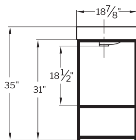
Round basin with apron and free standing frame codes Codes de cadre sur pied et bassin rond avec tablier
