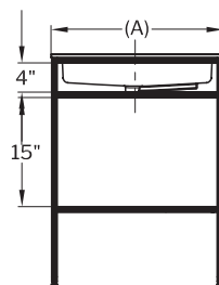
Square basin without apron and free standing frame codes Codes du bassin carré sans tablier et cadre sur pied
